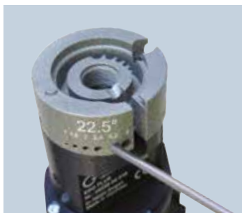
Affilatura di elettrodi: 4 angoli diversi, 6 diametri dell'elettrodo diversi
