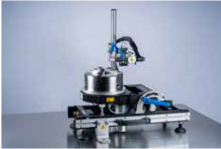
DVR M eingestellt für Vertikalschweißungen
